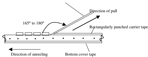
Fig. 4 Peeling Test
